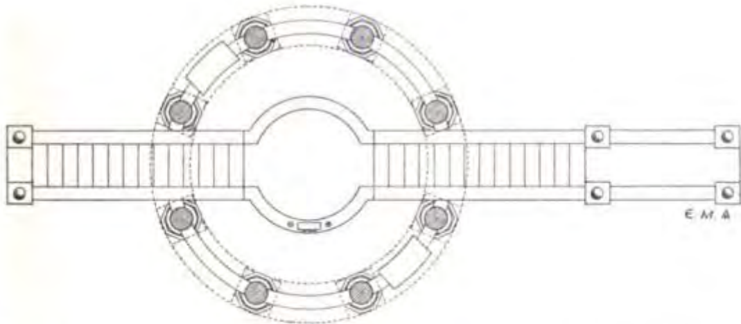
Σχ. 242. Ἀποκατάσταση τοῦ διαγράμματος τοῦ δευτέρου τῆς Ἀγίας Σοφίας Ἀμβωνος. Κλίμαξ=1/5.
