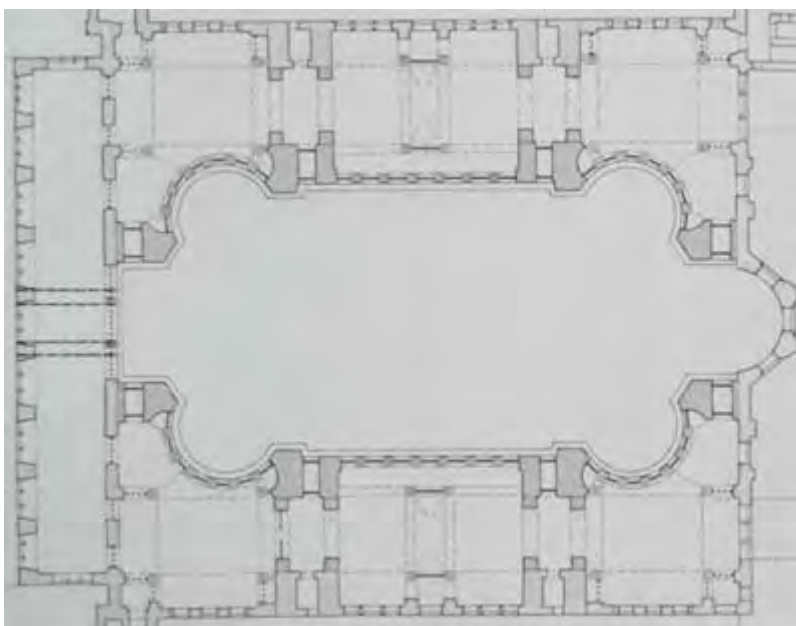
Εἰκ. 5-9. Ἡ ἐντυπωσιακὴ κάτοψις στὸ ἐπίπεδο τῶν ὑπερώων (gallery) στὴν Ἀγία Σοφία τοῦ Ἰουστινιανοῦ. 39
