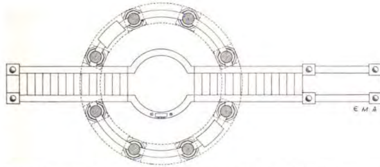
Σχ. 242. Ἀποκατάσταση τοῦ διαγράμματος τοῦ δευτέρου τῆς Ἁγίας Σοφίας Ἀμβωνος. Κλίμαξ=1/5.
