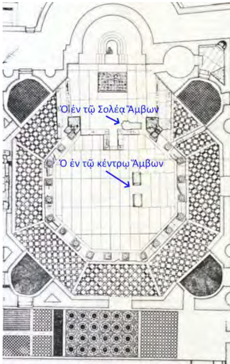
Εἰκ. 81-3. Ὁκταγωνικὴ Ἐκκλησίᾳ Φιλίππων, Στυλ. Πελεκανίδης, ΠΑΕ(1978), Μέρος ἐκ τοῦ Παρενθέτου Πίνακος Β'.
