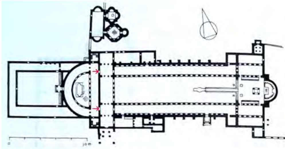
Εἰκ. 5-11. Κολοσσιαία Βασιλική τοῦ Ἀγίου Λεωνίδη (5 ος αἰ.) στὴν ἀρχαία Κόρινθο (λιμάνι Λεχαίου). 56, 57 (μῆκος ἀψίδος/κόγχης – νάρθηξ = π. 114 μ., χορδή ἀψίδος/κόγχης – νάρθηξ = π. 106 μ.)
